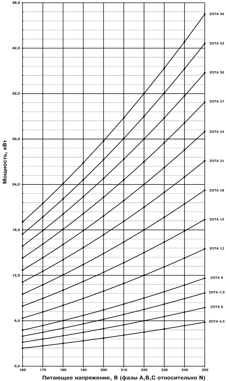
Рис.12 График изменения мощности электроводонагревателя в зависимости от питающего напряжения
