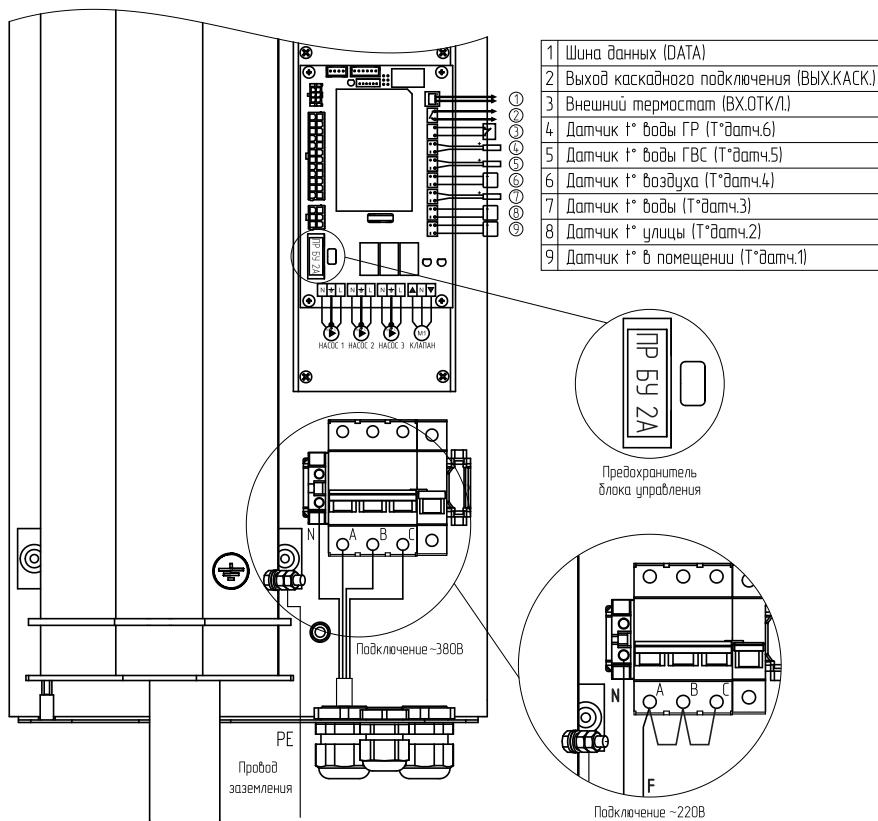
Рис. 3 Схема подключения электроводонагревателя
