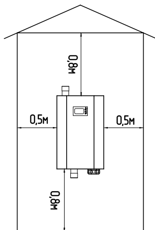
Рис. 4 Схема установки электроводонагревателя
